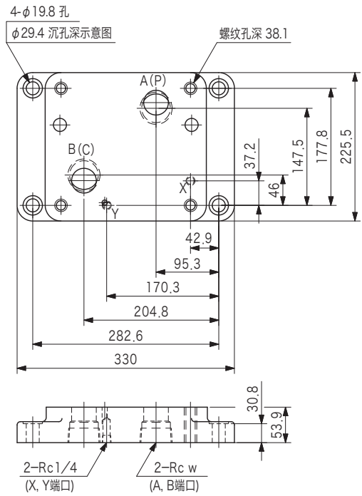
尺寸表
