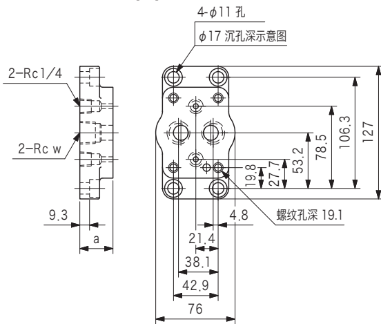
尺寸表
