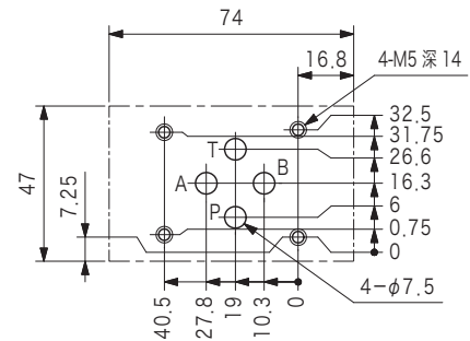
●安装面尺寸
