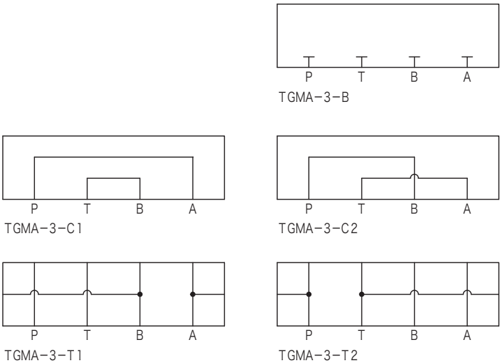
液压图形符号
