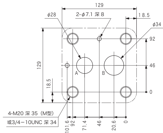
●安装面尺寸
