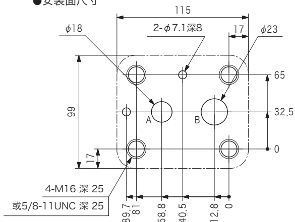
●安装面尺寸
