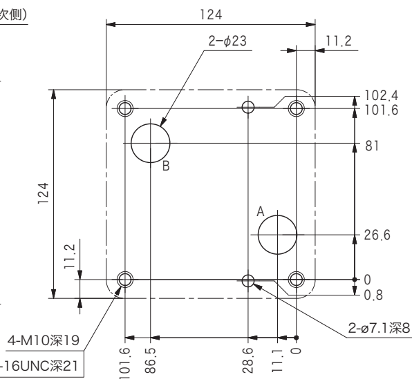
●安装面尺寸
