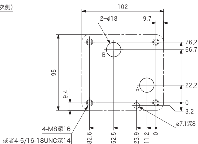
●安装面尺寸
