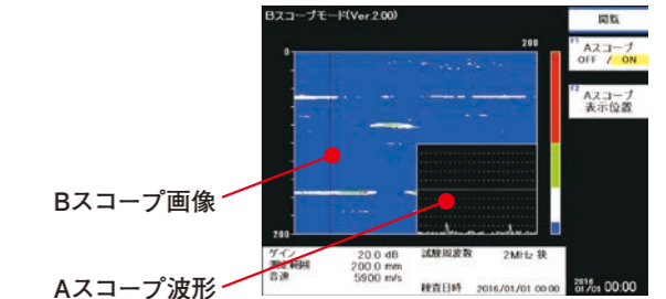
Aスコープ波形
