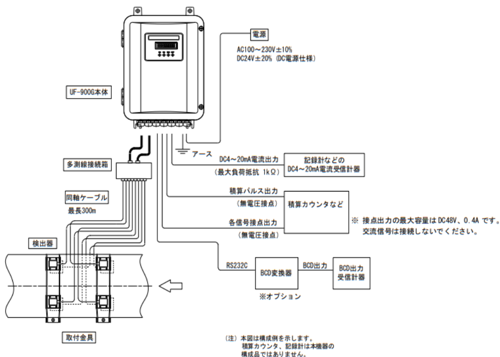
超音波流量計基本構成図 (UF-900G、4 測線)
