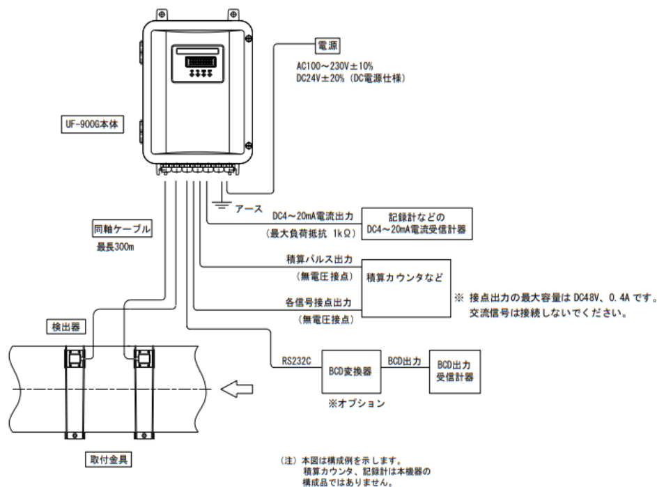
超音波流量計基本構成図 (UF-900G、1 測線)
