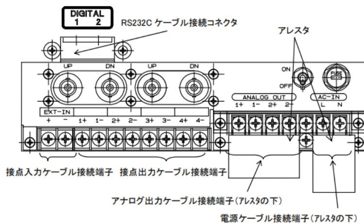
本体端子台付近図 (電源がAC仕様の場合)
