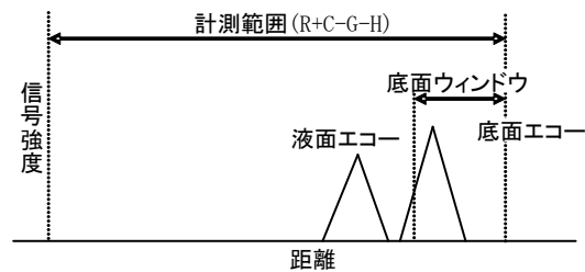
図 5. 4. 7 底面認識
