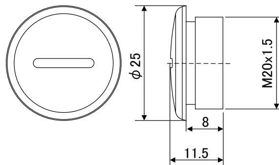
図 10. 7. 11 付属のブラインドプラグ (非防爆仕様用)
