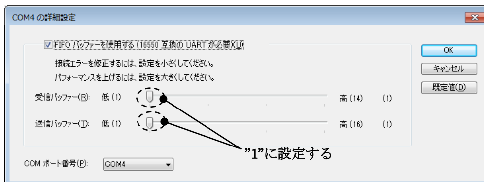
図 6. 1. 2 COM ポート設定
