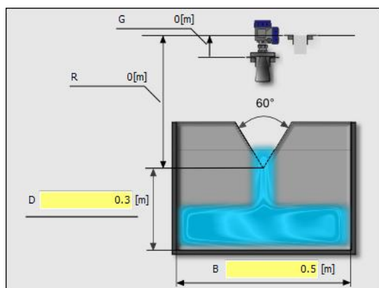
60° 三角堰
