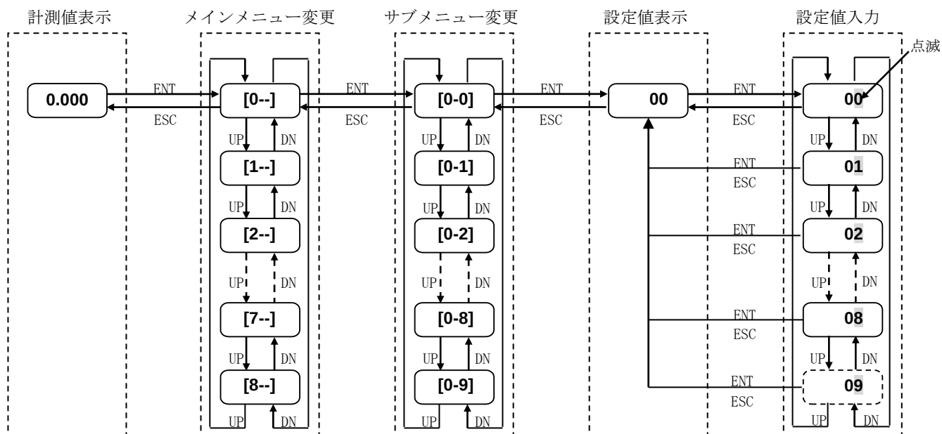
図 5. 2. 1 メニュー遷移
