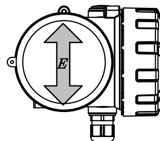
図 2. 7. 1 電波の偏波面
