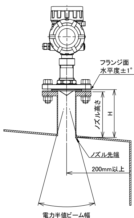
図 2. 2. 2 プロセスシールアンテナの取り付け例
