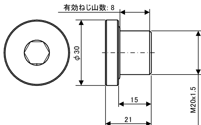
図10. 7. 10 付属のブラインドプラグ （国内防爆 耐圧/本安組合せ防爆仕様用）
