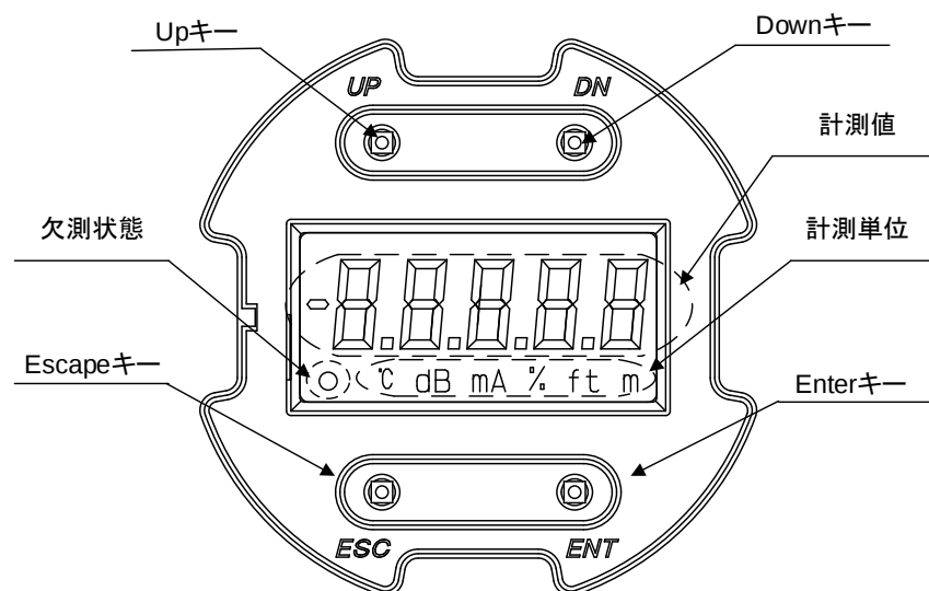
図 5. 1. 2 LCD とキー
