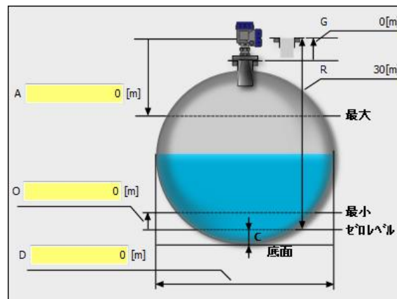
球形タンク
