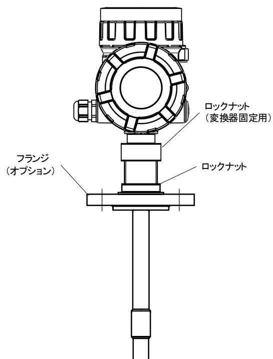
図 2. 1 0. 1 2 フランジの固定 (ロッドアンテナ/25A-10K フランジ)
