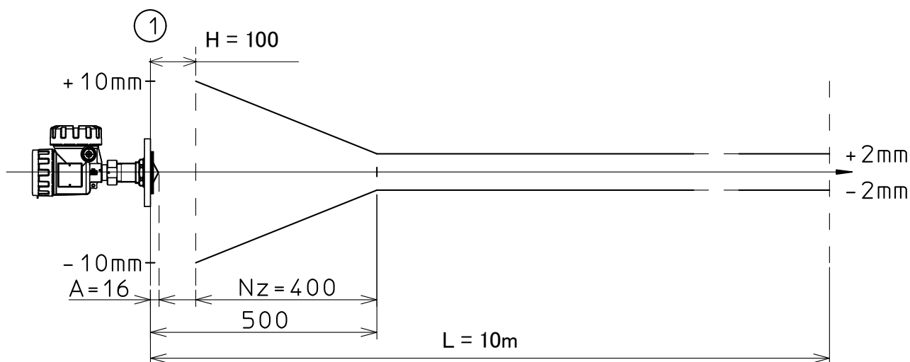
図 10. 1. 4 2B プロセスシールアンテナ最大計測誤差
