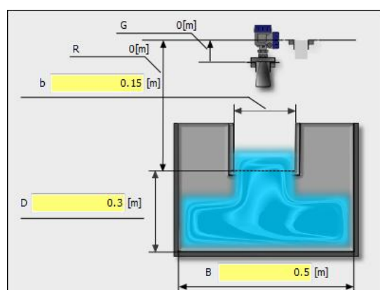
四角堰
