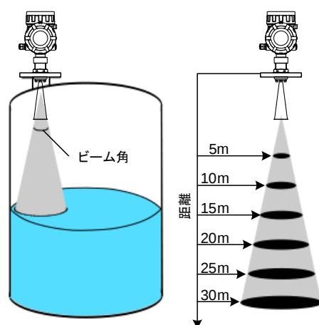
図 2. 3. 1 ビーム角と距離
