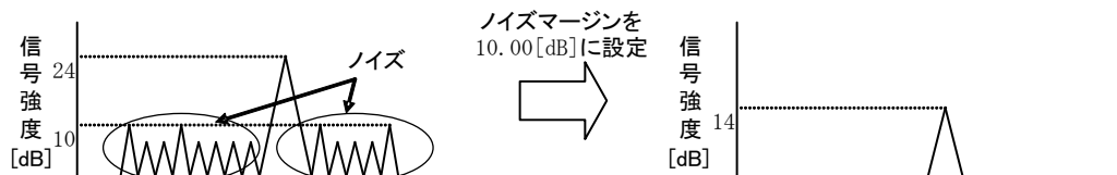
図 5. 4. 4 ノイズマージン
