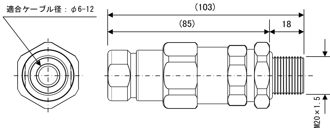
図10. 7. 9 付属の耐圧防爆構造パッキン式ケーブルグランド （国内防爆 耐圧/本安組合せ防爆仕様用）
