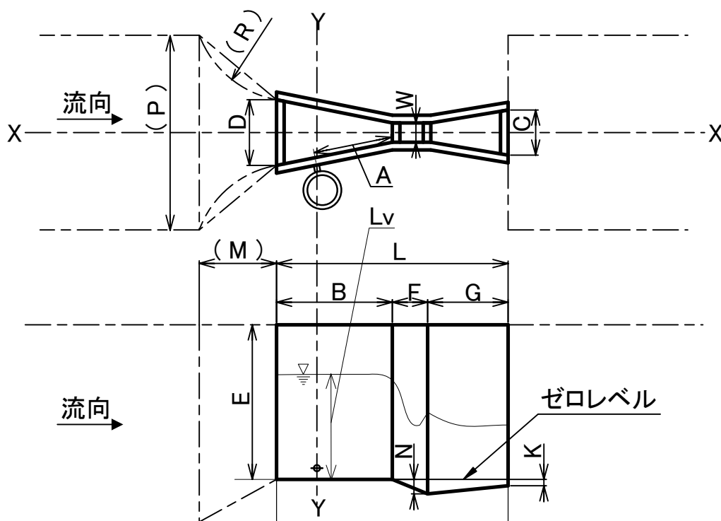
図 6. 3. 6 パーシャルフリューム
