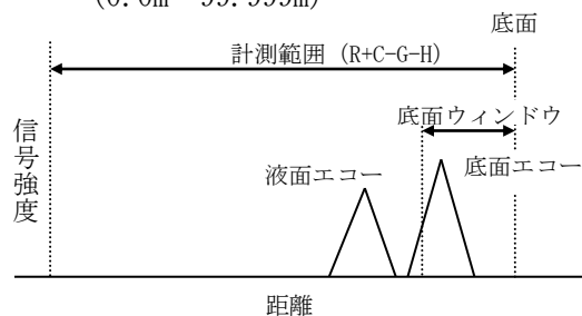
図 6. 6. 8 底面認識
