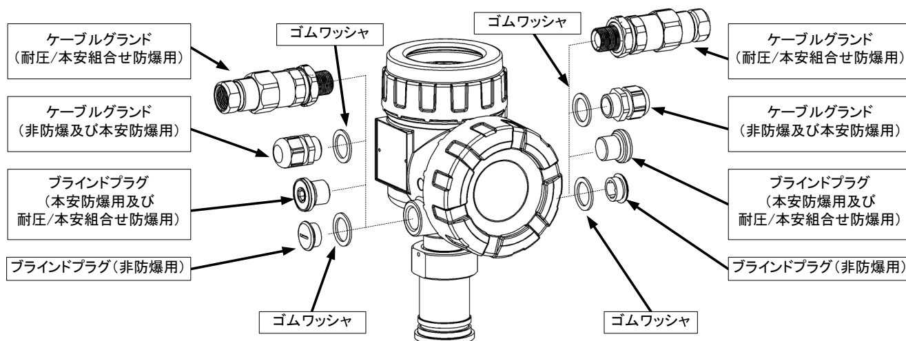
図 3. 1. 2 各部名称
