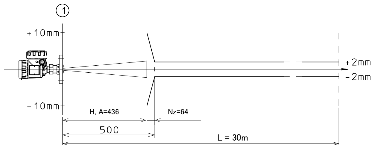
図 10. 1. 2 4B コーンアンテナ最大計測誤差
