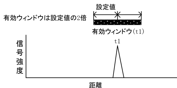
図 6. 6. 6 有効ウィンドウ
