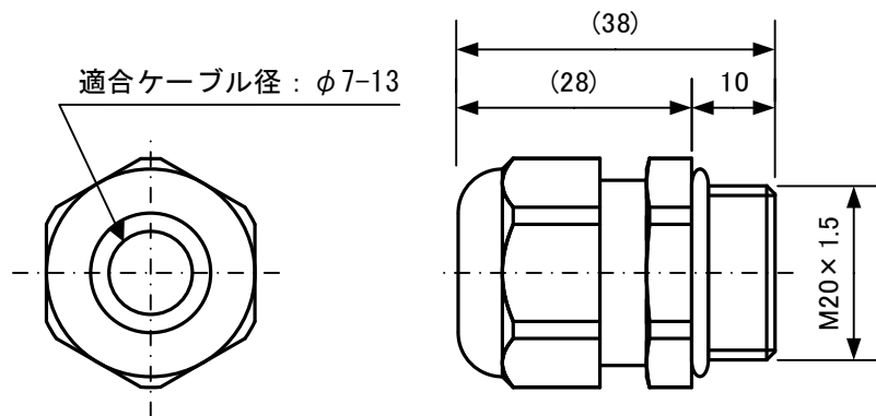
図10. 7. 8 付属のケーブルグランド（非防爆仕様， 国内防爆 本質安全防爆仕様用）
