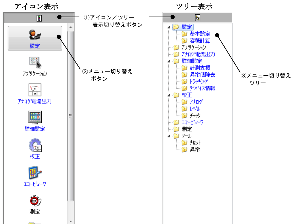
図 6. 1. 15 メニュー選択部の表示
