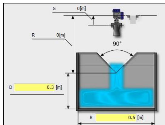
90° 三角堰
