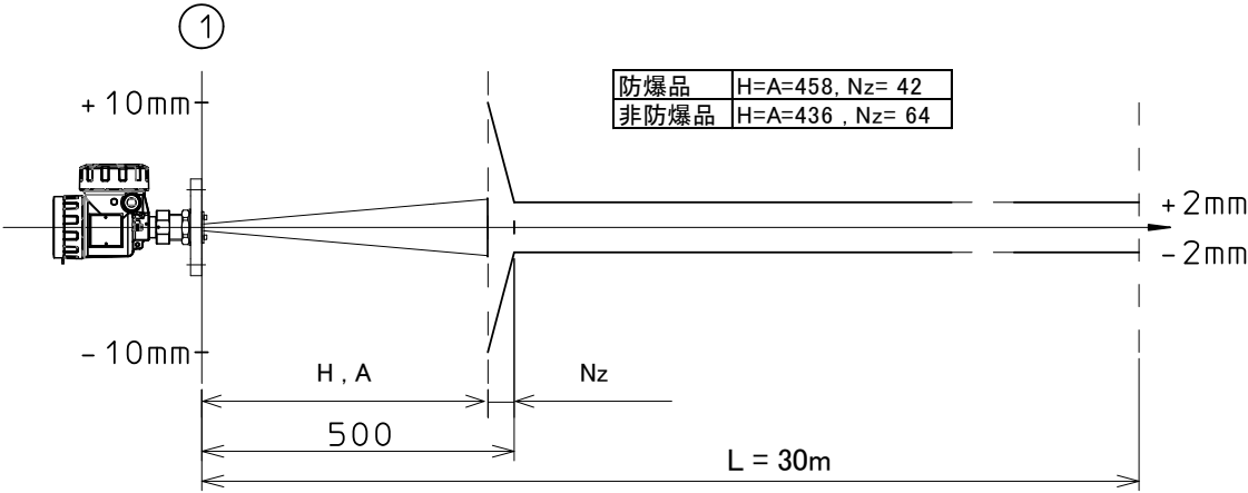
4B コーンアンテナ最大計測誤差
