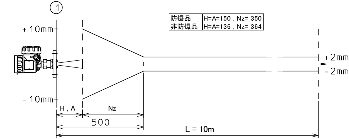
2B コーンアンテナ最大計測誤差
