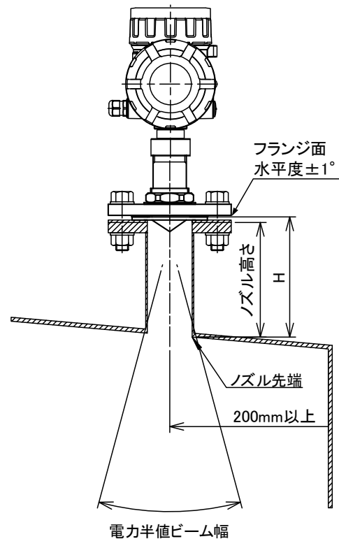
プロセスシールアンテナ
