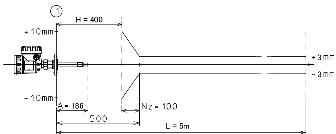
1B ロッドアンテナ最大計測誤差
