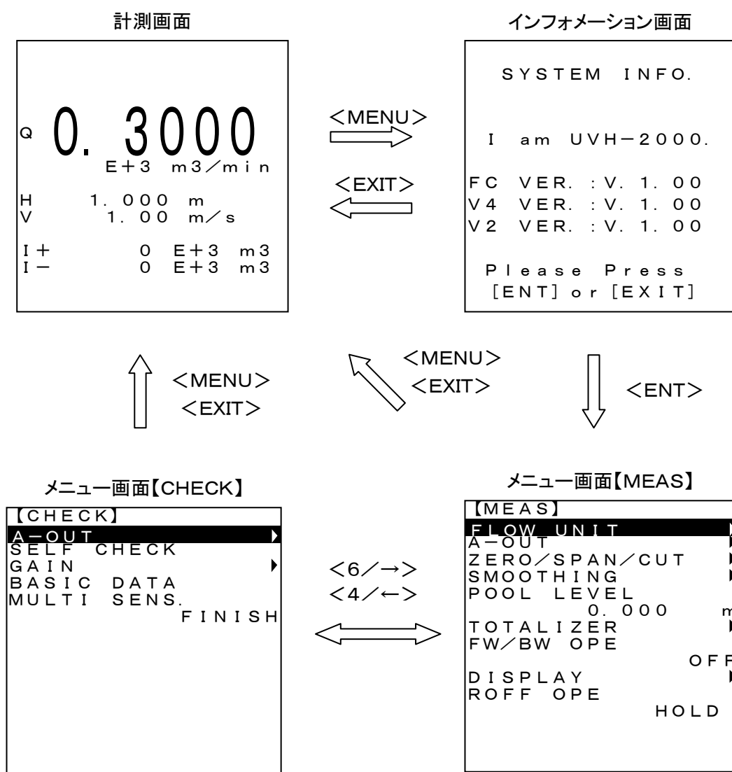
図4-4-1 計測画面とメニュー画面
