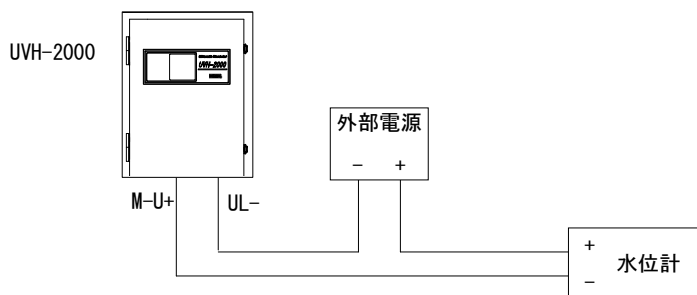
図5-3 外部電源接続図
