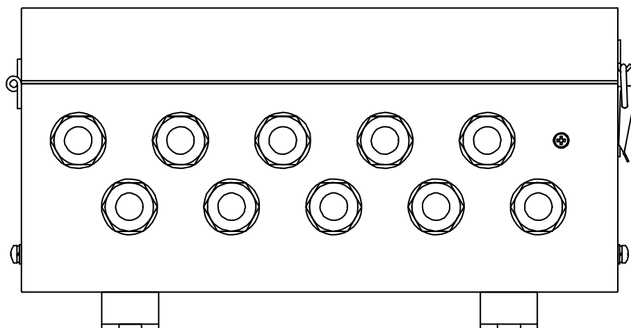
図5-2 本体ケース下面
