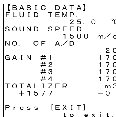
図4-9-2 b BASIC DATA表示画面例
