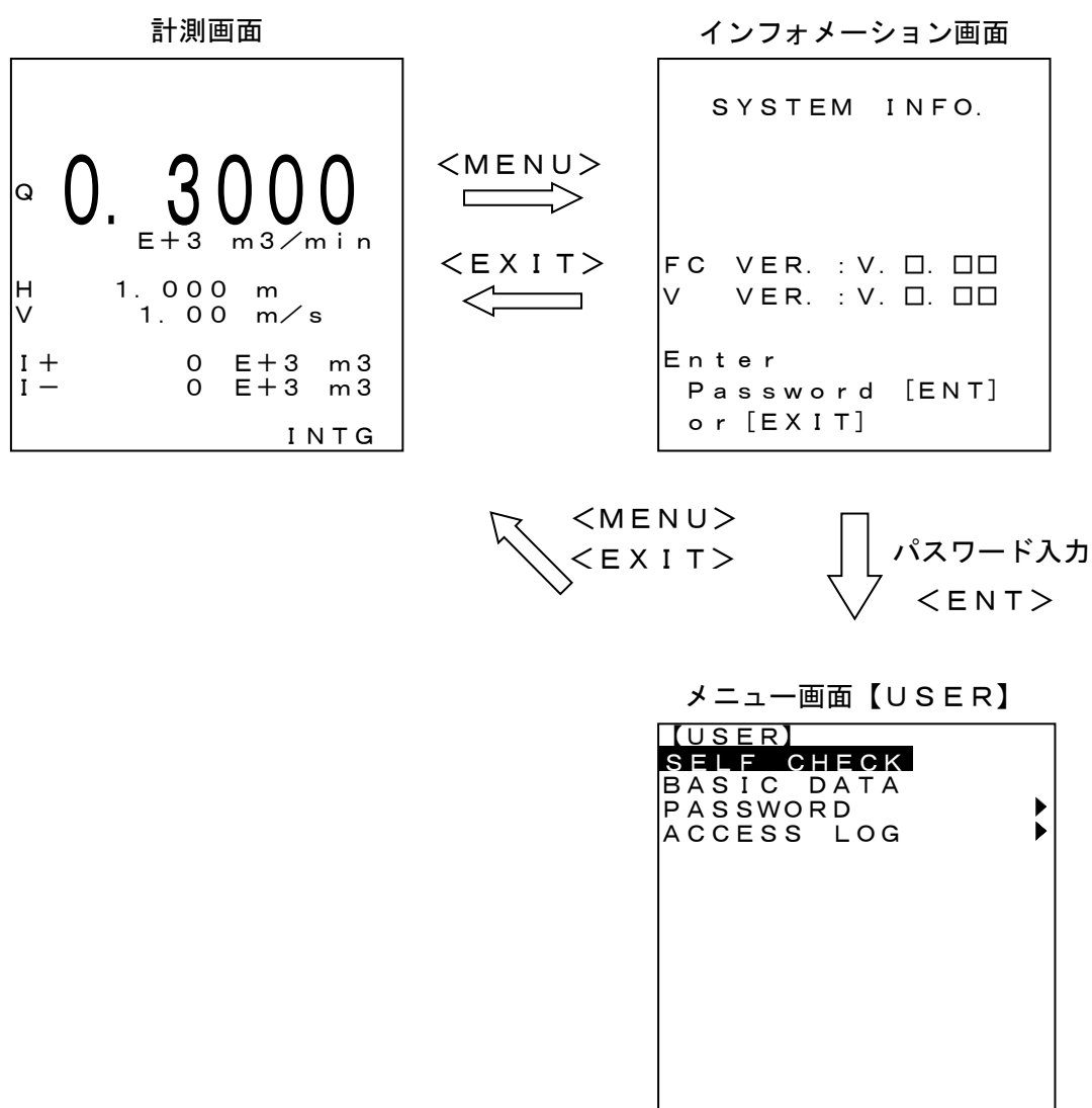
図4-4 計測画面とメニュー画面
