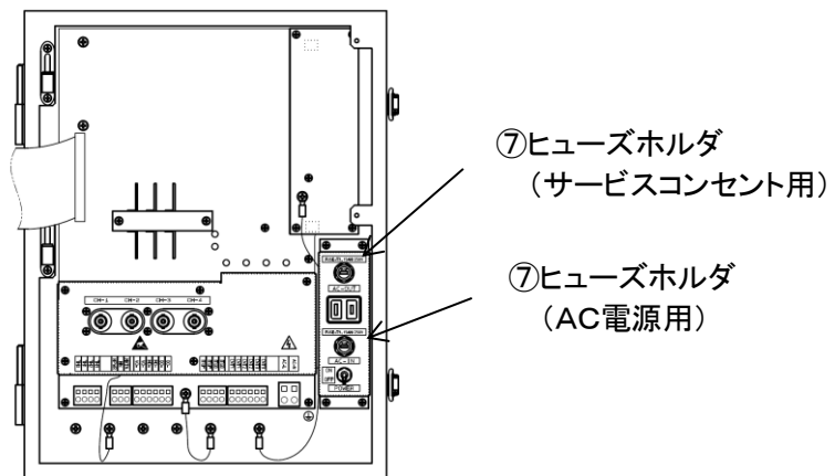
図3-3 パネルが開いている状態
