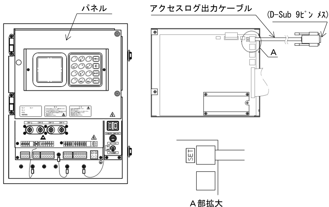
図4. 9. 4a ケーブル接続図
