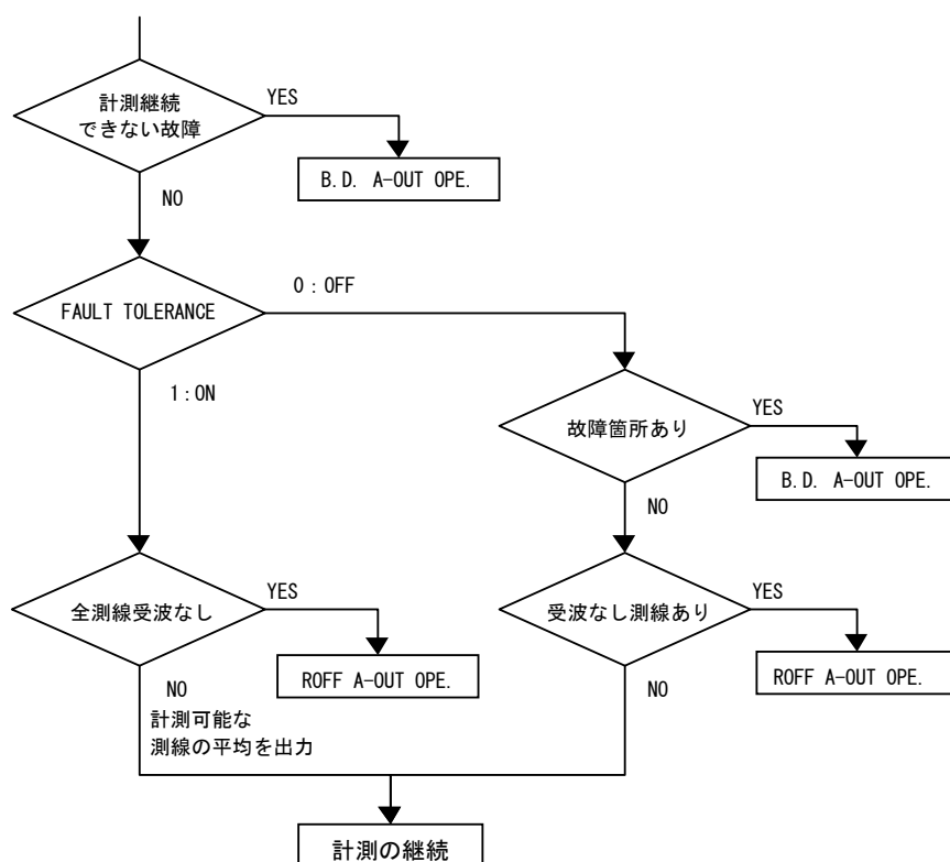
図 4-4 ; 計測異常時遷移図
