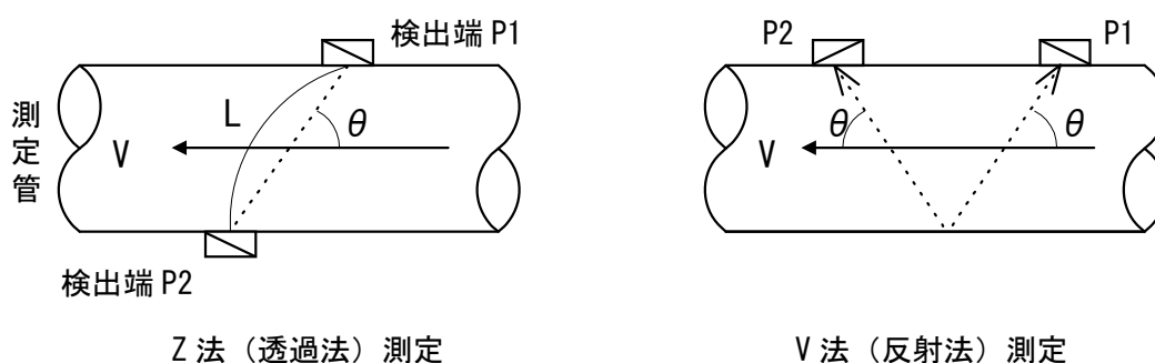
図 7-2；測定方式
