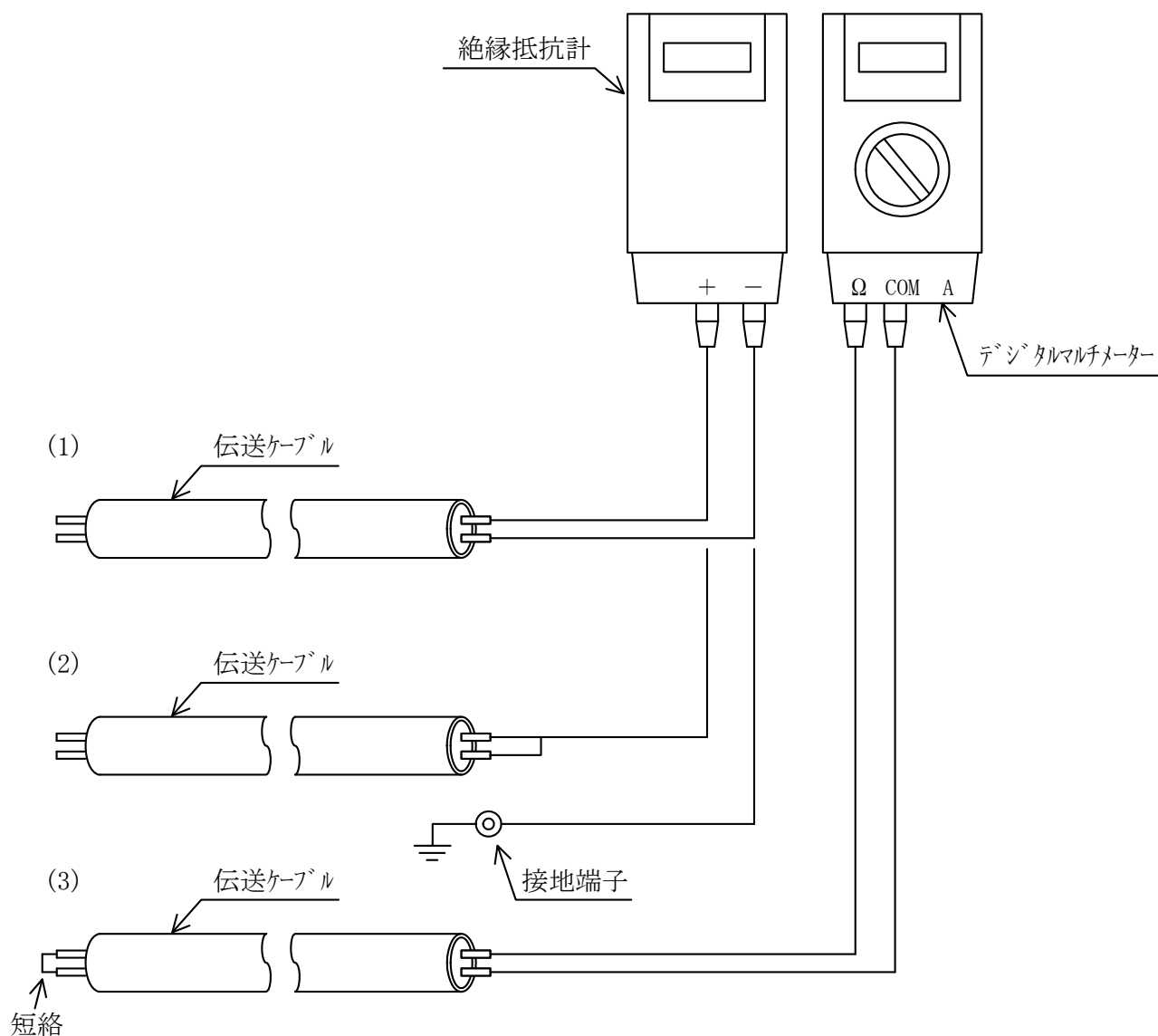
図 31 伝送ケーブルの点検
