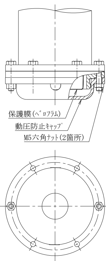
図 19 PL-200C 型検出器受圧部
