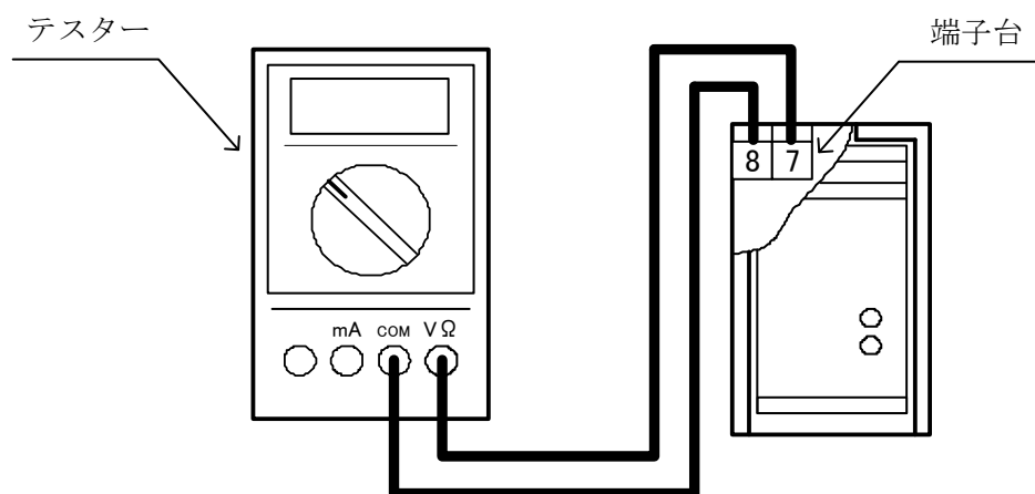
図 25 変換器への供給電圧の測定
