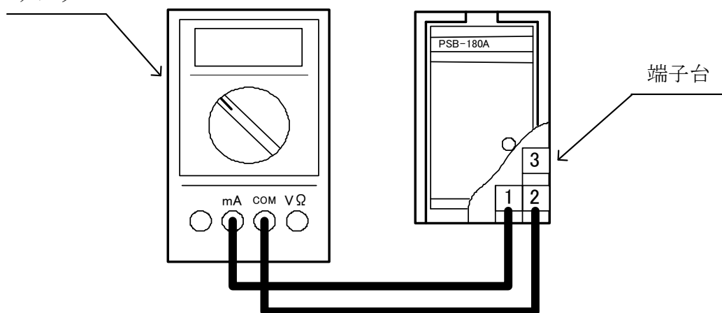
図 27 変換器出力電流の測定 (PSB-180□型)
