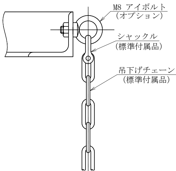
図2 チェーンの固定方法
