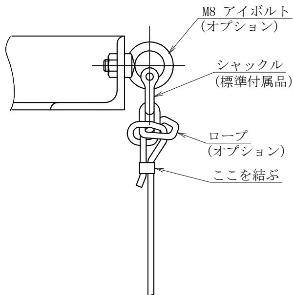
図3 ロープの固定方法
