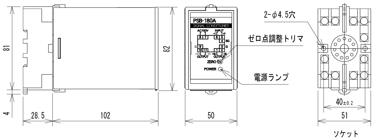
端子番号図
