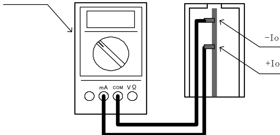
図 28 変換器出力電流の測定 (PSB-180□型)
