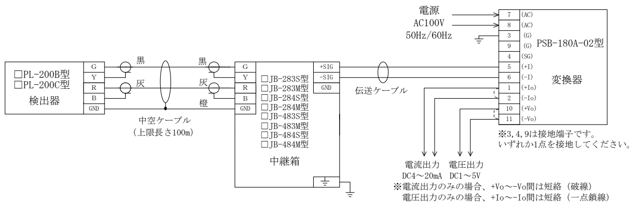
図 10 機器間結線図（AC 用）
