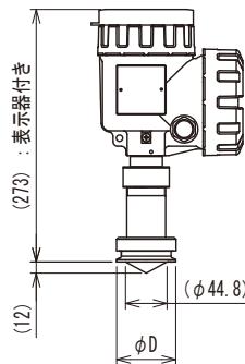
4Bコーンアンテナ
