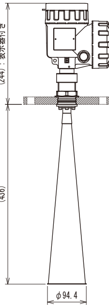
4Bコーンアンテナ
