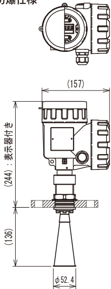
2Bコーンアンテナ
