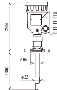
1Bロッドアンテナ
