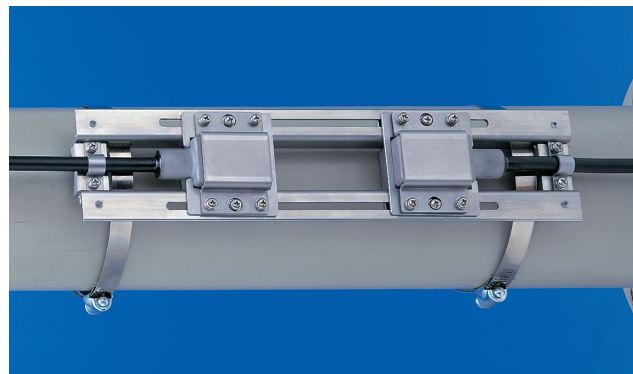
検出器 (UFM-400G)
