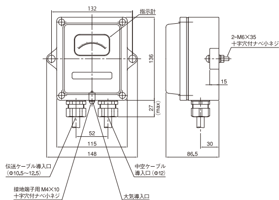
中継箱 JB-483M
