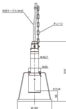
検出器 PL-200B
