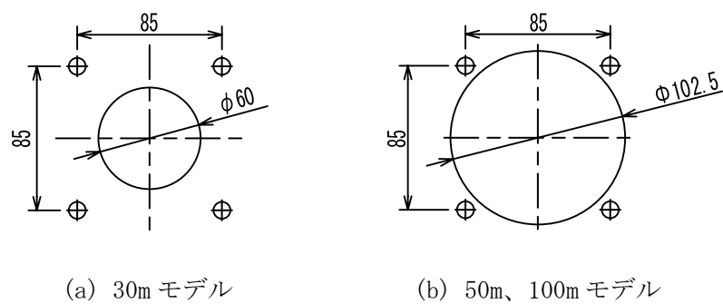
図 5.4.6 取付寸法参考図
