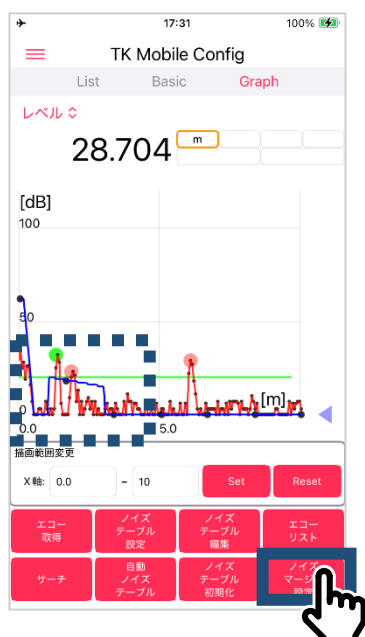
図 4. 4. 3. 8 ノイズマージンの設定
