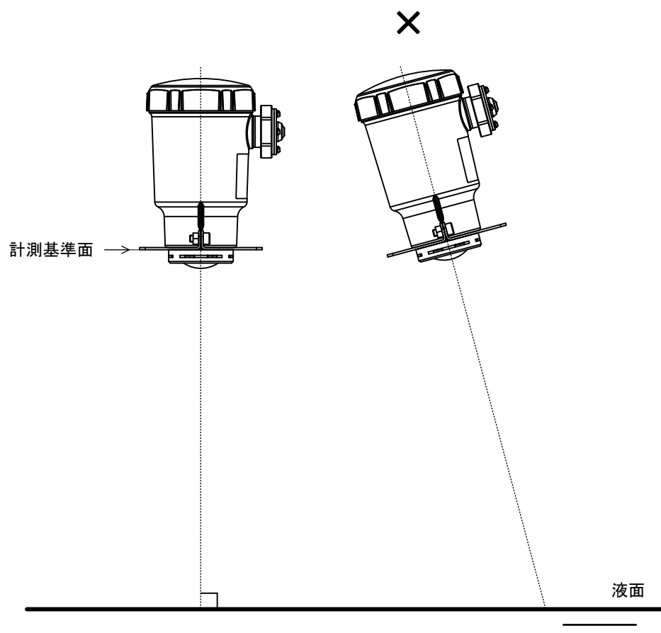
図2.2.2 取付角度
