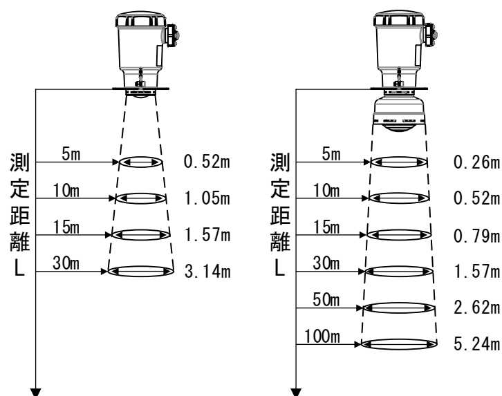
図2.3.1 ビーム径
