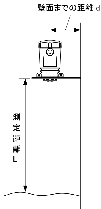
図2.4.1 壁面距離
