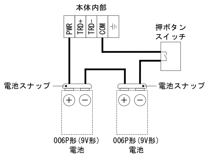
図 3.1.1.4 内部結線
