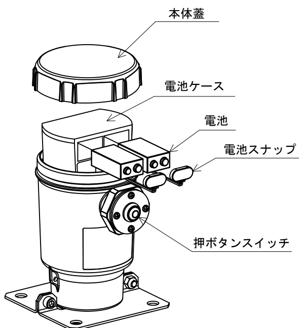
図 3.1.1.1 押ボタンスイッチ操作および電池取付手順
