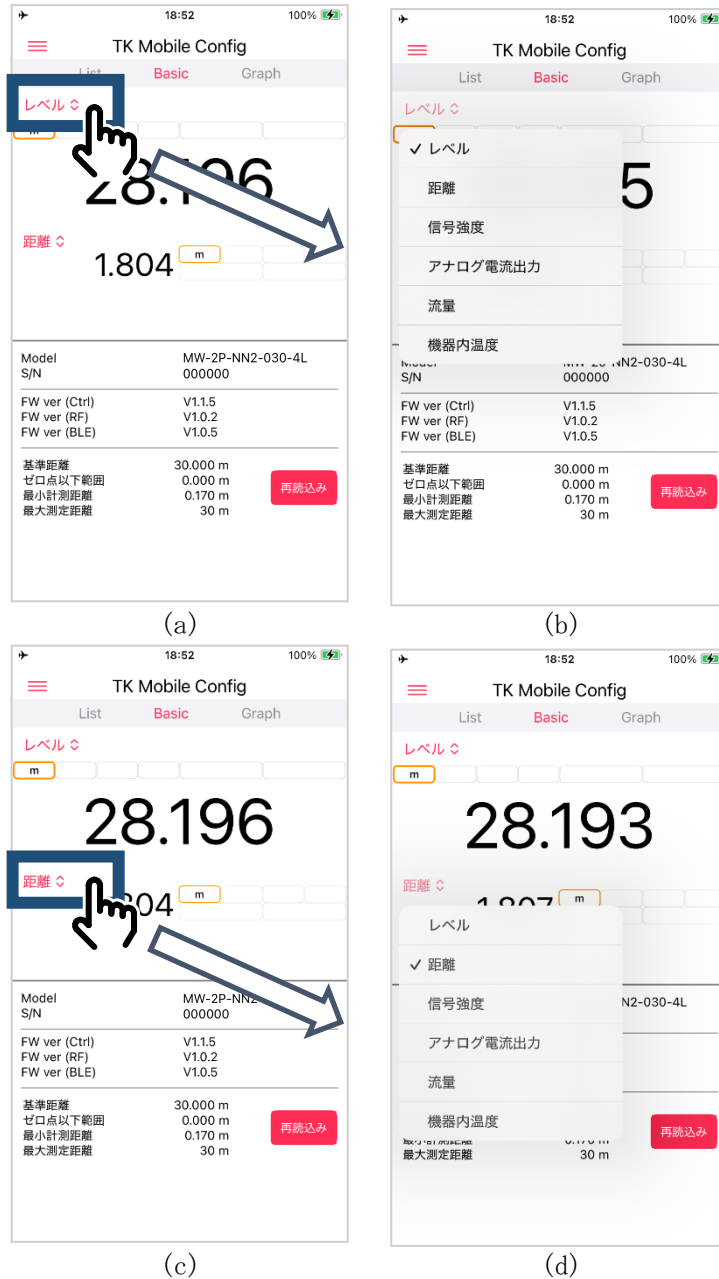
図 4.4.2.1 BASIC 画面(例)
