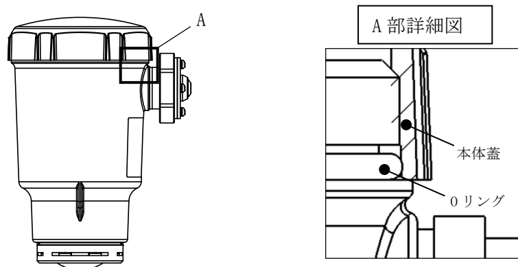
図 3.1.2.1 本体蓋の取付
