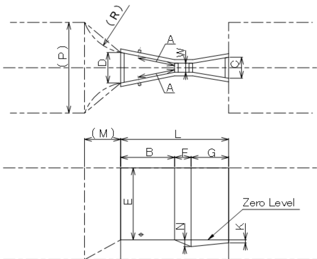
図 4.5.3.3 パーシャルフリューム
