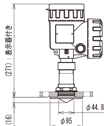
2Bプロセスシールアンテナ
