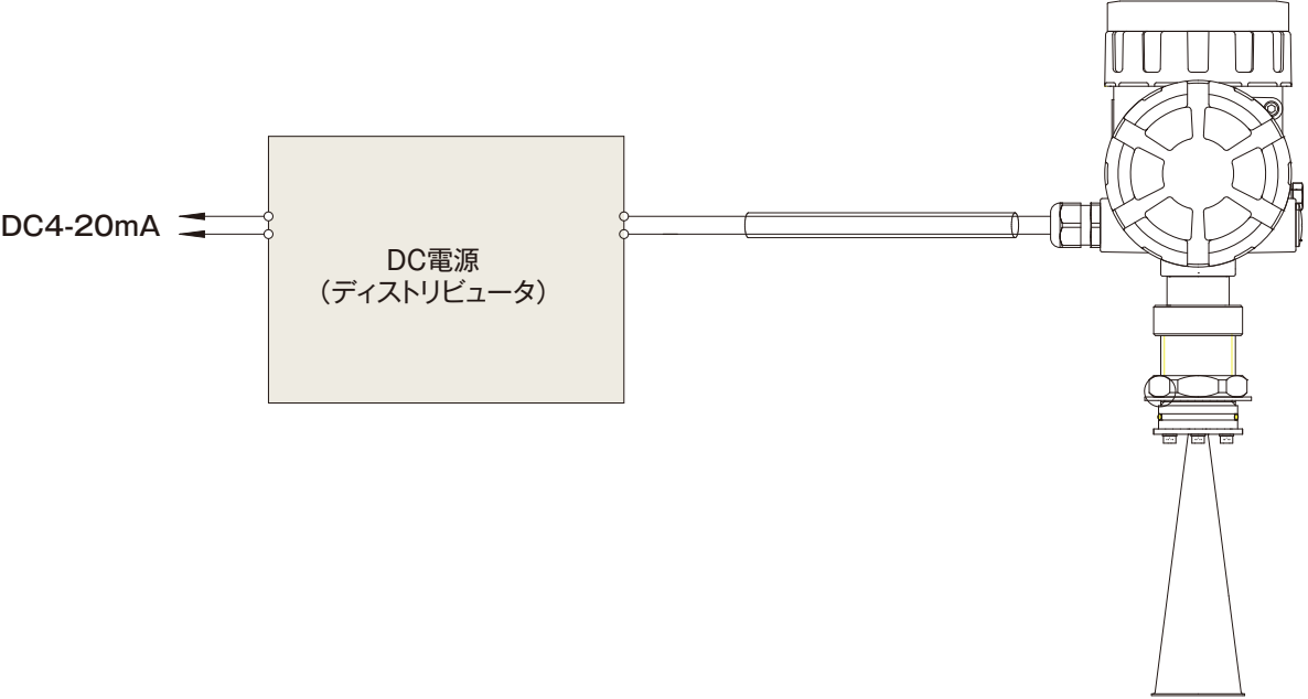
製品接続例
