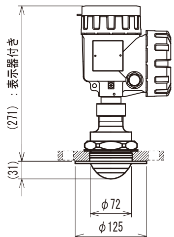
3Bプロセスシールアンテナ
