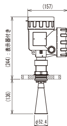
2Bコーンアンテナ
