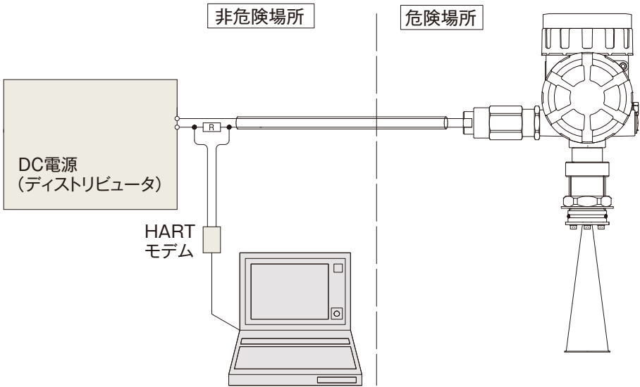
耐圧/本安組合せ防爆製品接続例
