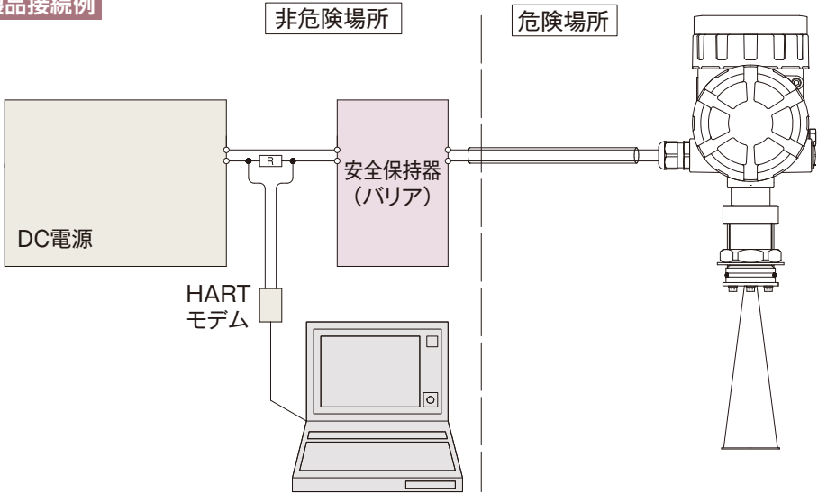
本質安全防爆製品接続例
