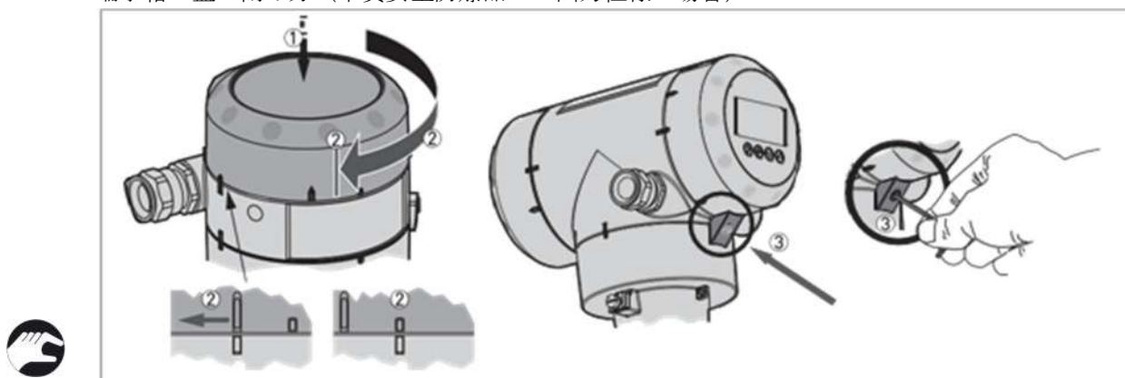
図 3-3： 端子箱の蓋の閉め方（Ex i の 1 出力仕様の場合）
