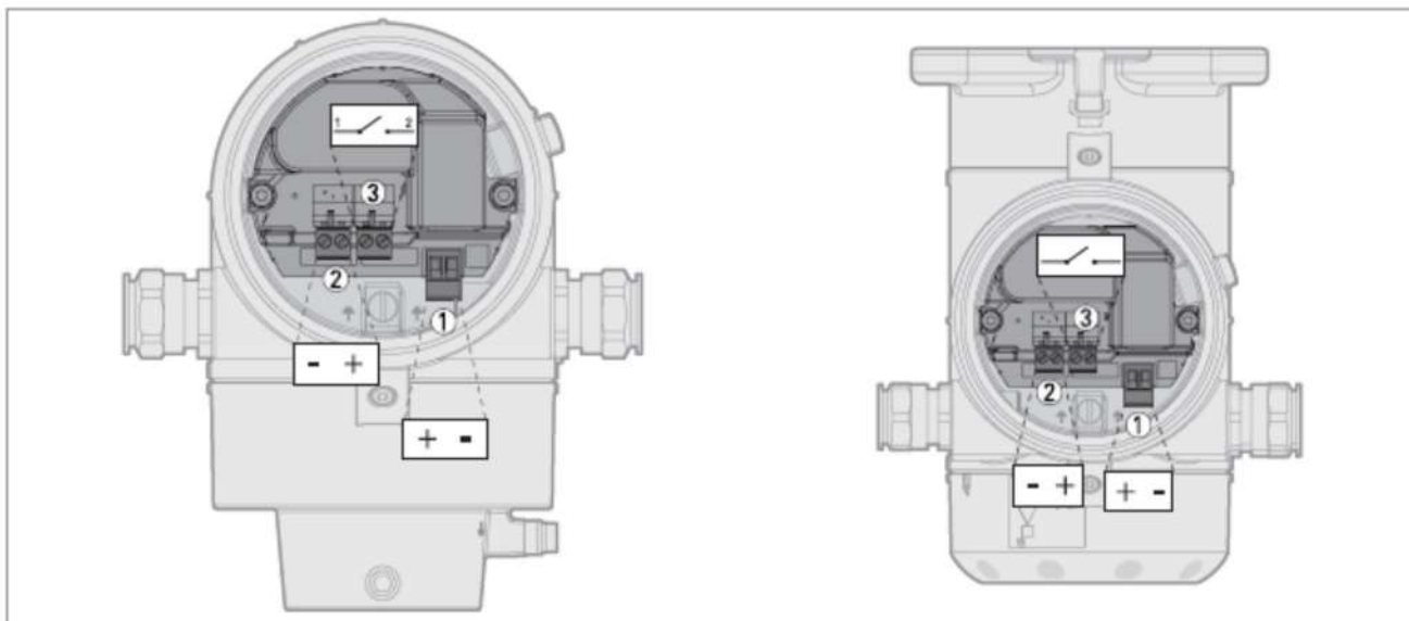
図 3-8：電流出力＋接点出力の端子配置
