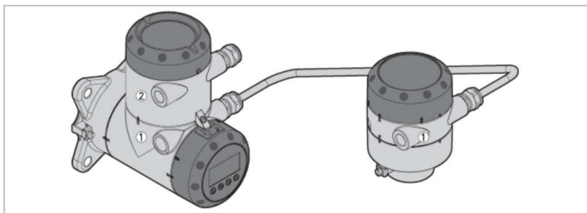
図 3-11： 分離形 Ex ia/db- 及び Ex ia/tb-認定機器のハウジング構成
