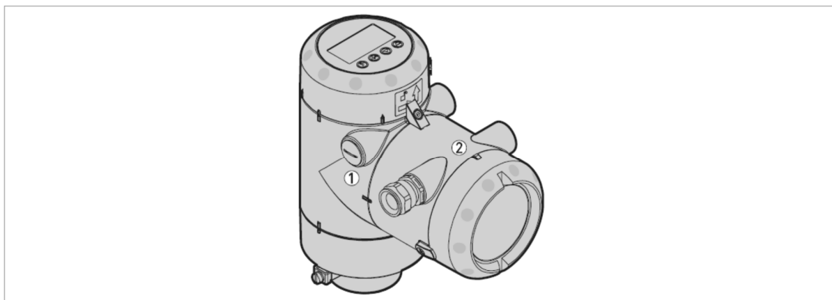
図 3-10： 一体形ハウジング Ex ia/db- 及び Ex ia/tb-認定機器のハウジング構成
