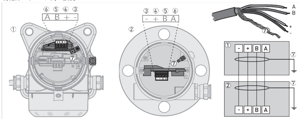
図 3-16: 分離コンバータハウジングとプローブハウジングの接続
