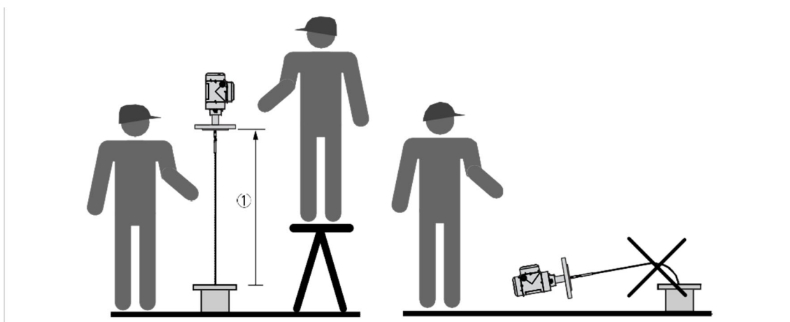
図 2-32 : フレキシブルプローブの設置
