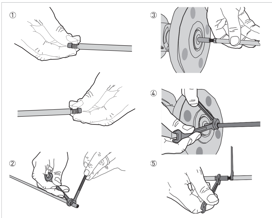
図 2-24 : セグメントリジッドシングルプローブの組付け
