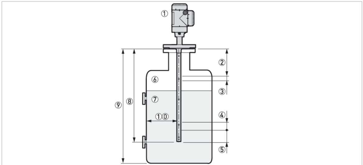
図 7-9:計測可能範囲(コアキシャル)
