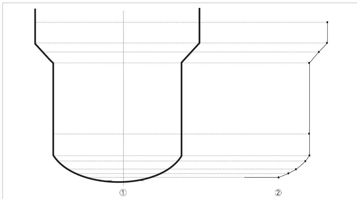
図 5-8: 容量、質量テーブルの入力ポイント
