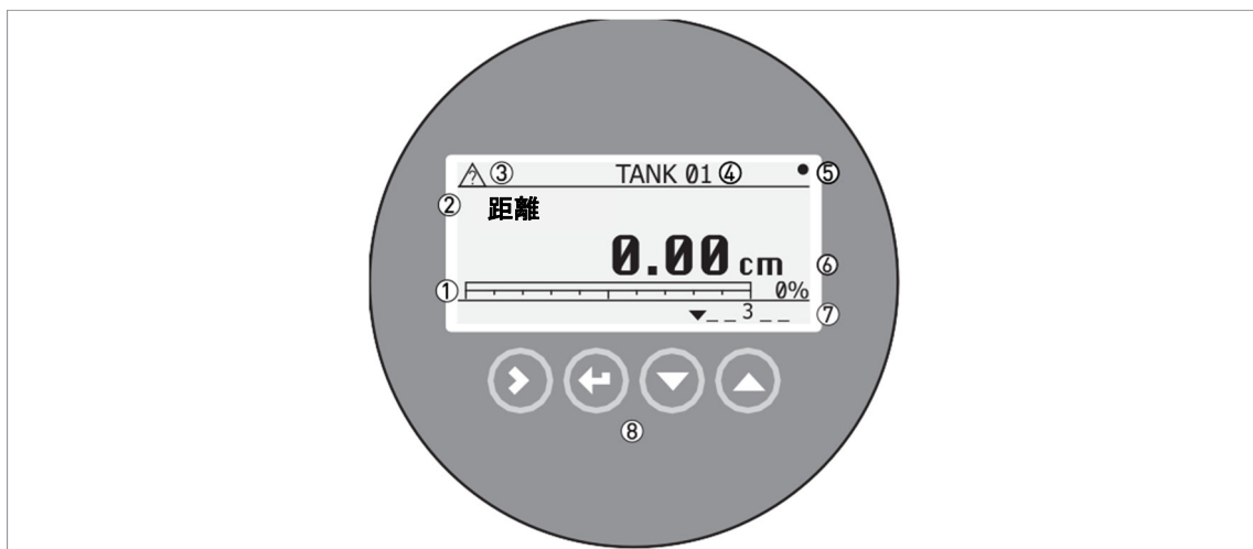
図 4-1：測定モード時の本体表示ユニットレイアウト
