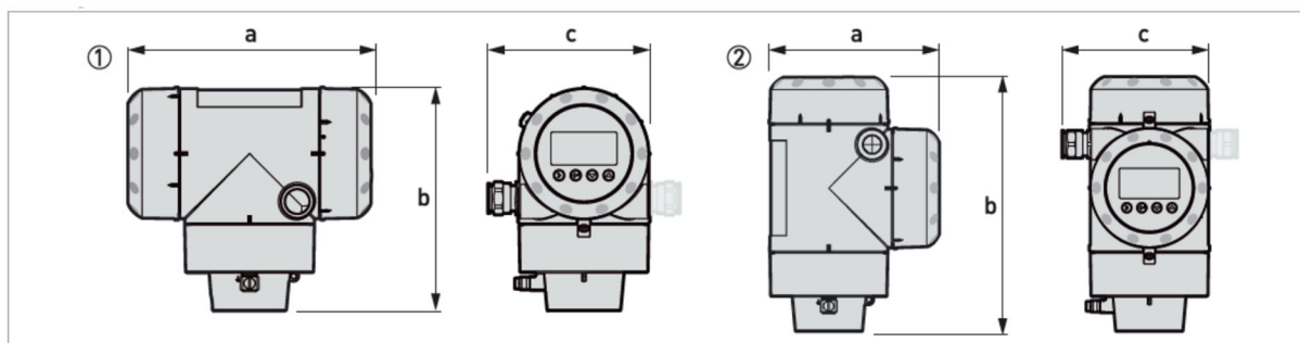
図 7-11: 一体形ハウジング(GWS-7200C)
