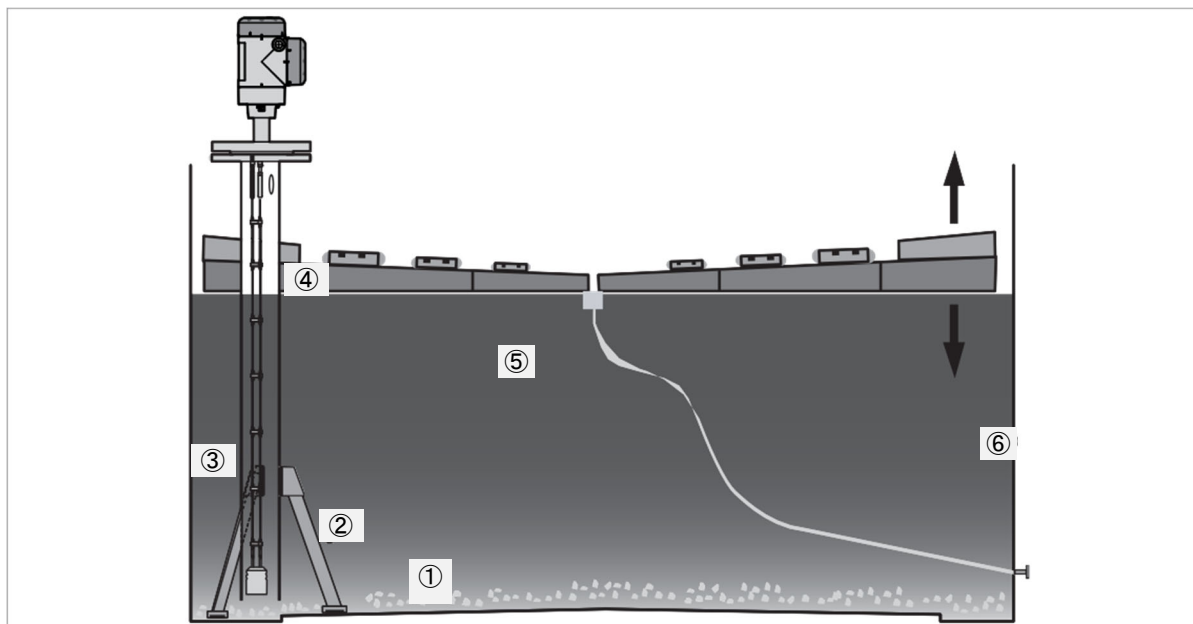
図 2-17 : フローティングルーフタンクの設置方法
