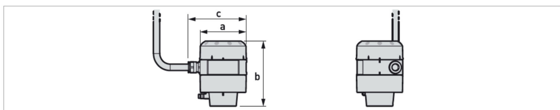
図 7-13: 分離コンバータハウジング(GWS-7200F)/プローブハウジング
