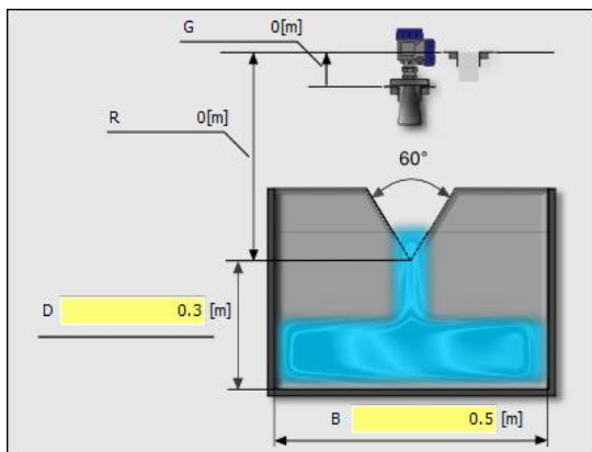
60° 三角堰
