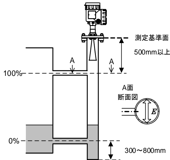
図 2. 8. 2 バイパス管を使用した設置
