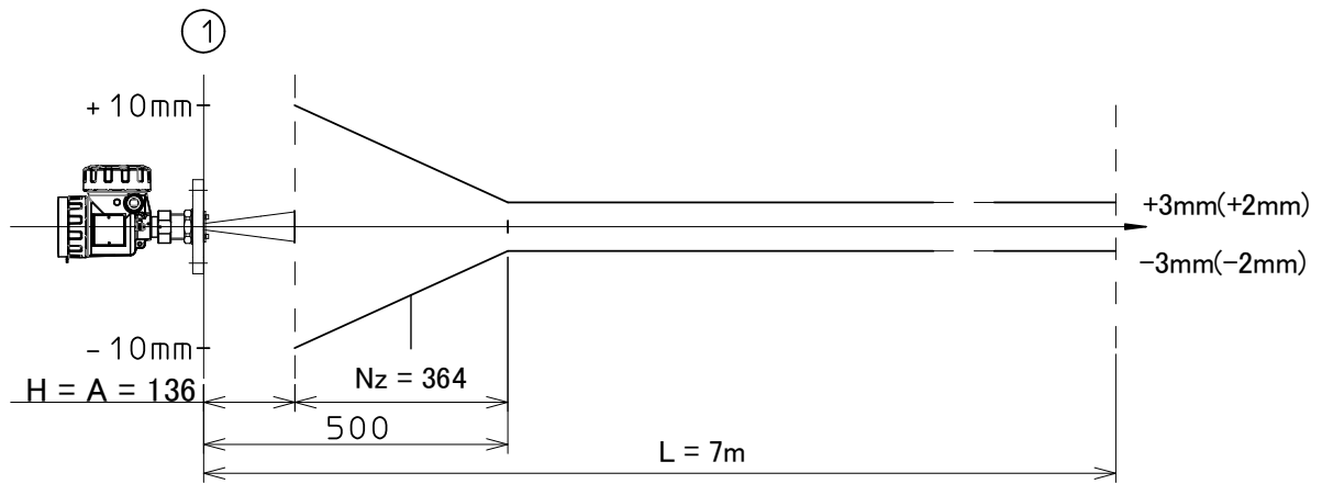
図 10. 1. 1 2B コーンアンテナ最大計測誤差
