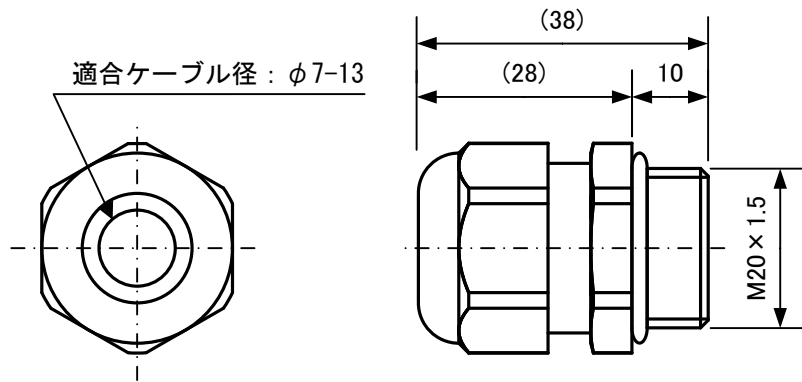
図10. 7. 6 ケーブルグランド
