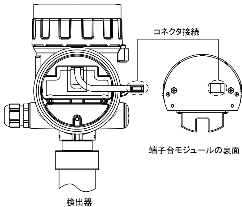
図 8. 4. 2 端子台モジュールの取り付け
