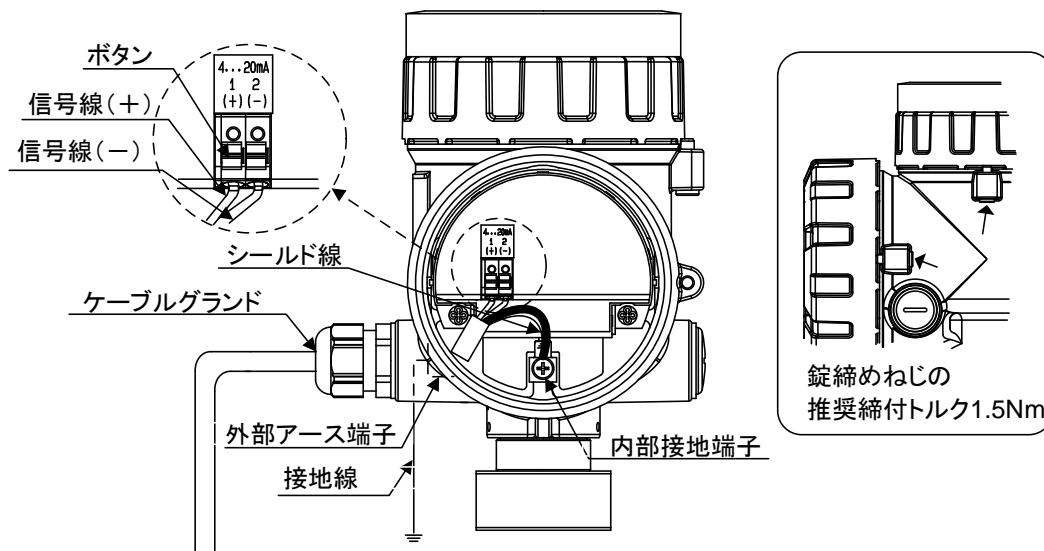
図3. 1. 1 結線図
