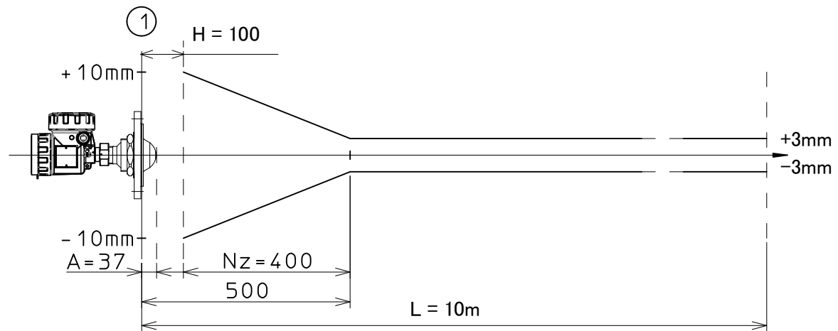
図 10. 1. 6 4B プロセスシールアンテナ最大計測誤差
