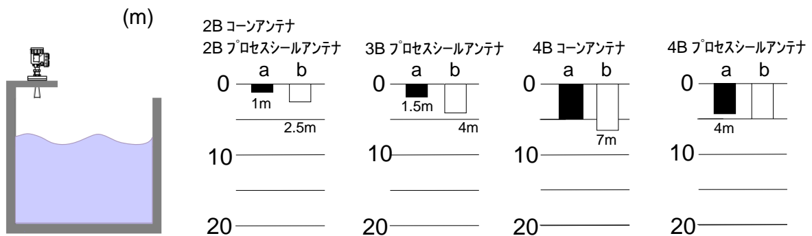
図 10. 1. 9 乱れた液面を持つタンクの測定距離
