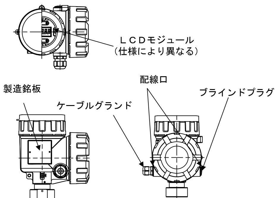
図 1. 2. 1 変換器外形図
