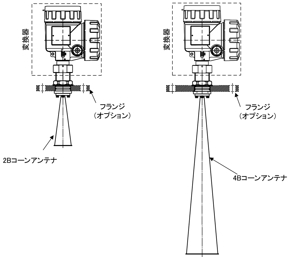
図 1. 2. 2 コーンアンテナ接続図
