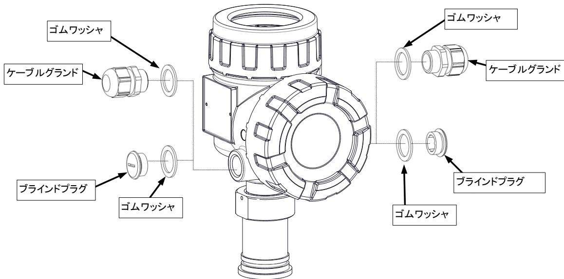
図 3. 1. 2 各部名称
