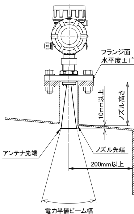
図 2. 2. 1 コーンアンテナの取り付け例
