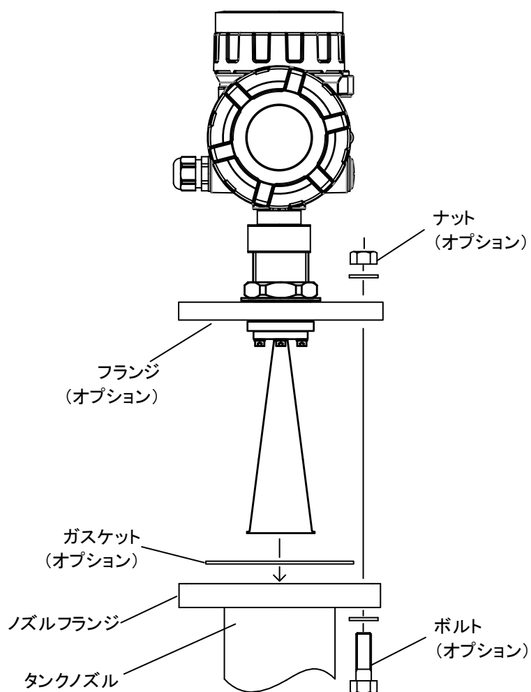
図 2. 10. 4 レベル計のタンクへの取り付け
