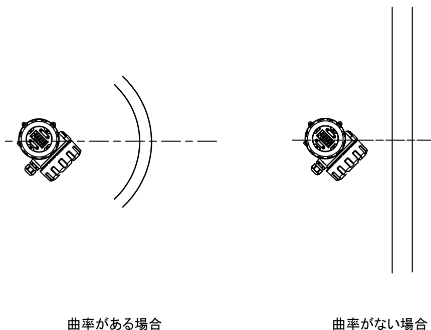
図 2. 7. 7 円筒タンクへの設置
