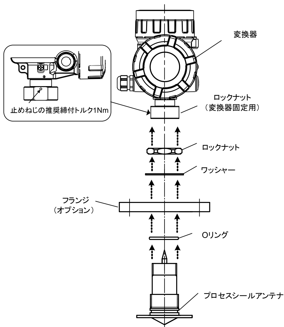
図 2. 10. 6 変換器とプロセスシールアンテナの固定
