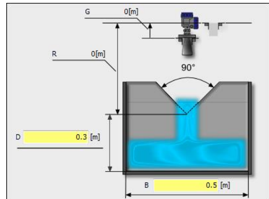
90° 三角堰
