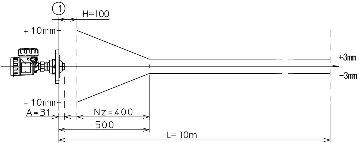
図 10. 1. 5 3B プロセスシールアンテナ最大計測誤差
