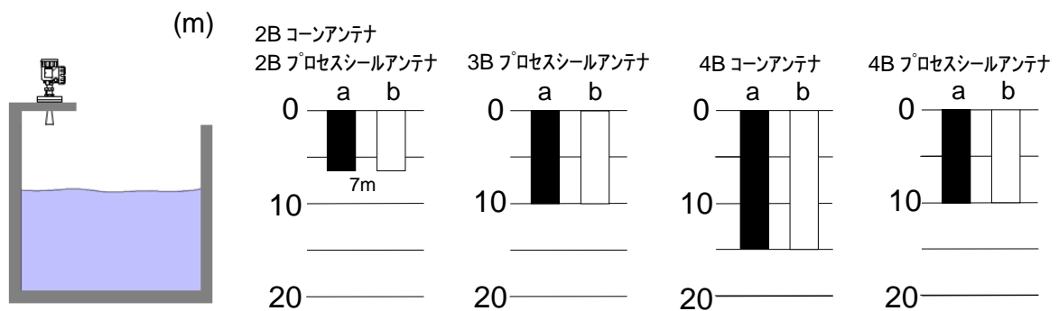
図 10. 1. 8 静かな液面を持つタンクの測定距離
