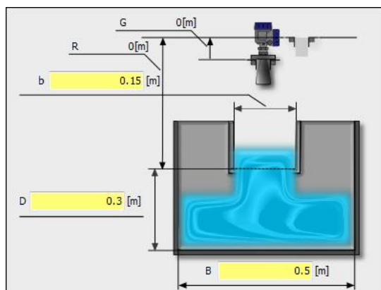
四角堰
