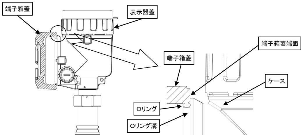
図 3. 1. 3 端子箱蓋の組付 (表示器蓋も同様)
