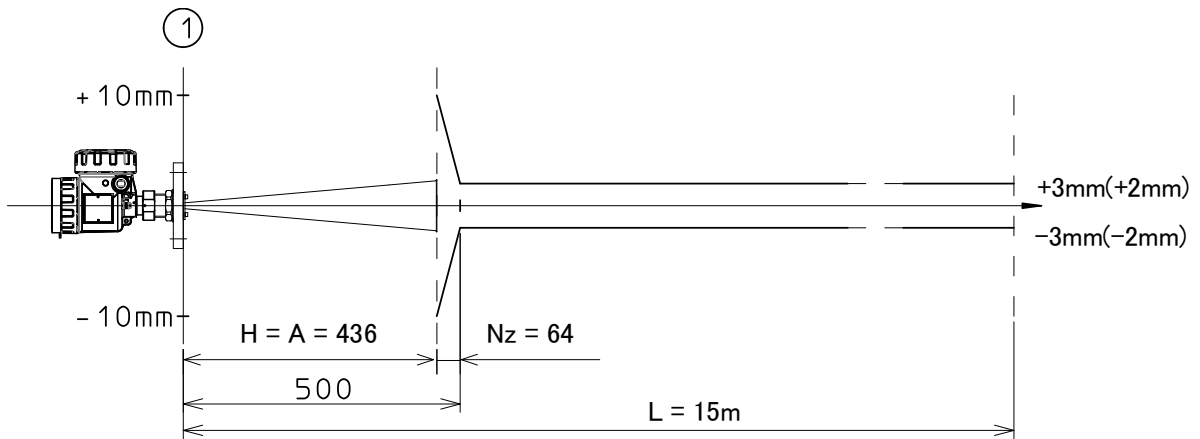
図 10. 1. 2 4B コーンアンテナ最大計測誤差
