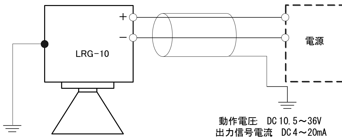
図 3. 1. 4 接続例
